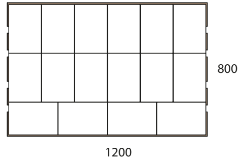
widok pierwszej warstwy palety first layer view
